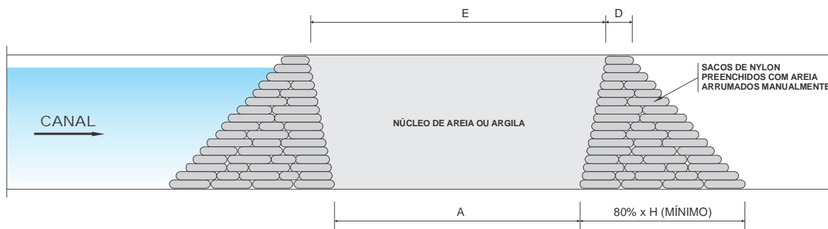
ENSECADEIRA TIPO 1 (Sacos de Nylon e Núcleo de Areia ou Argila)
