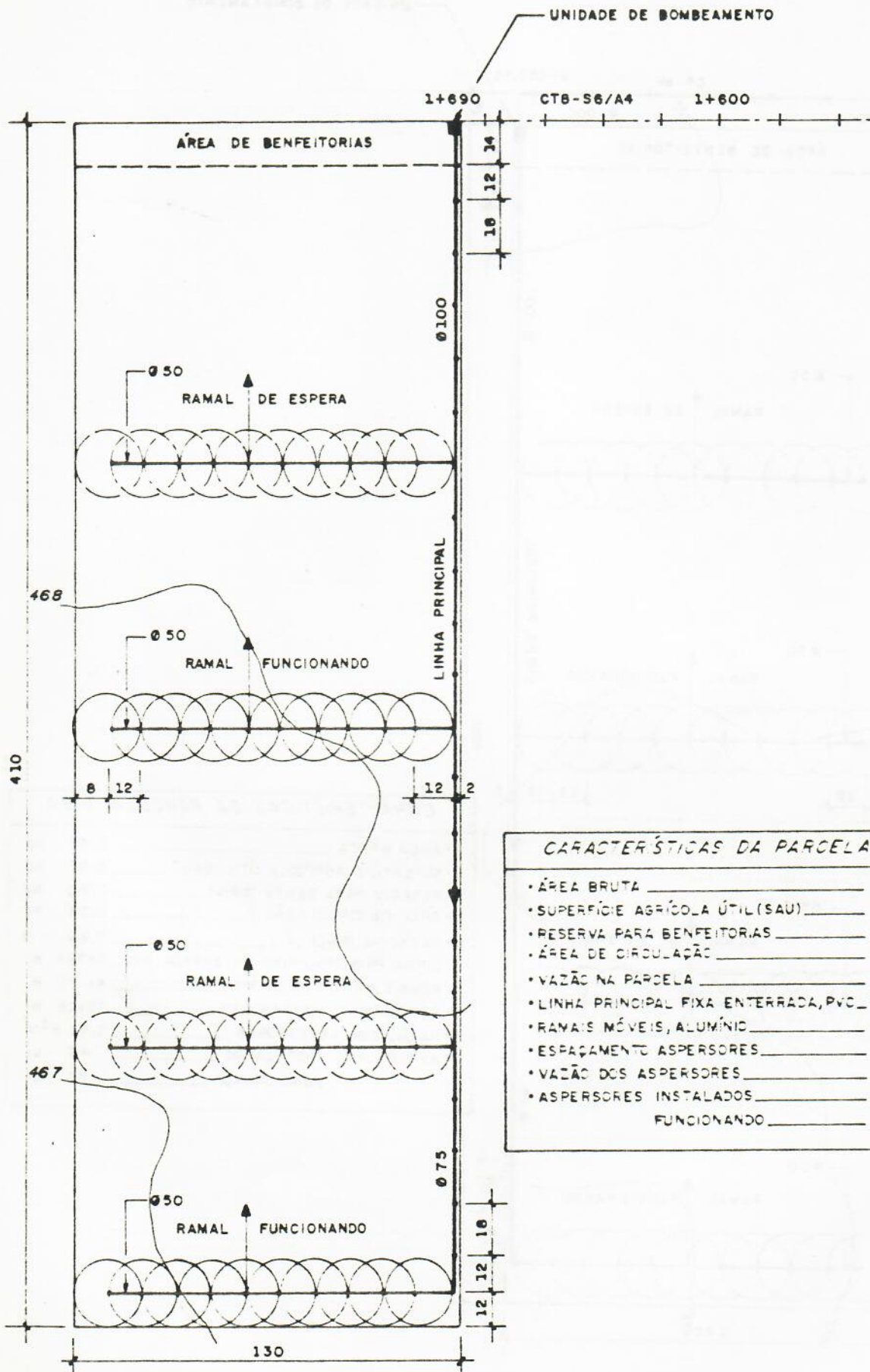
Fig. 877 REDE PARCELAR
