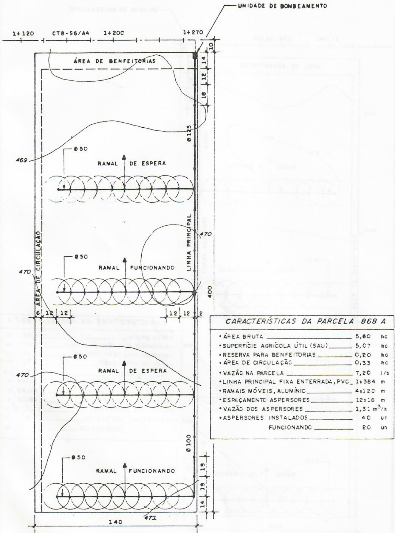
Fig. 5.25 REDE PARCELAR
