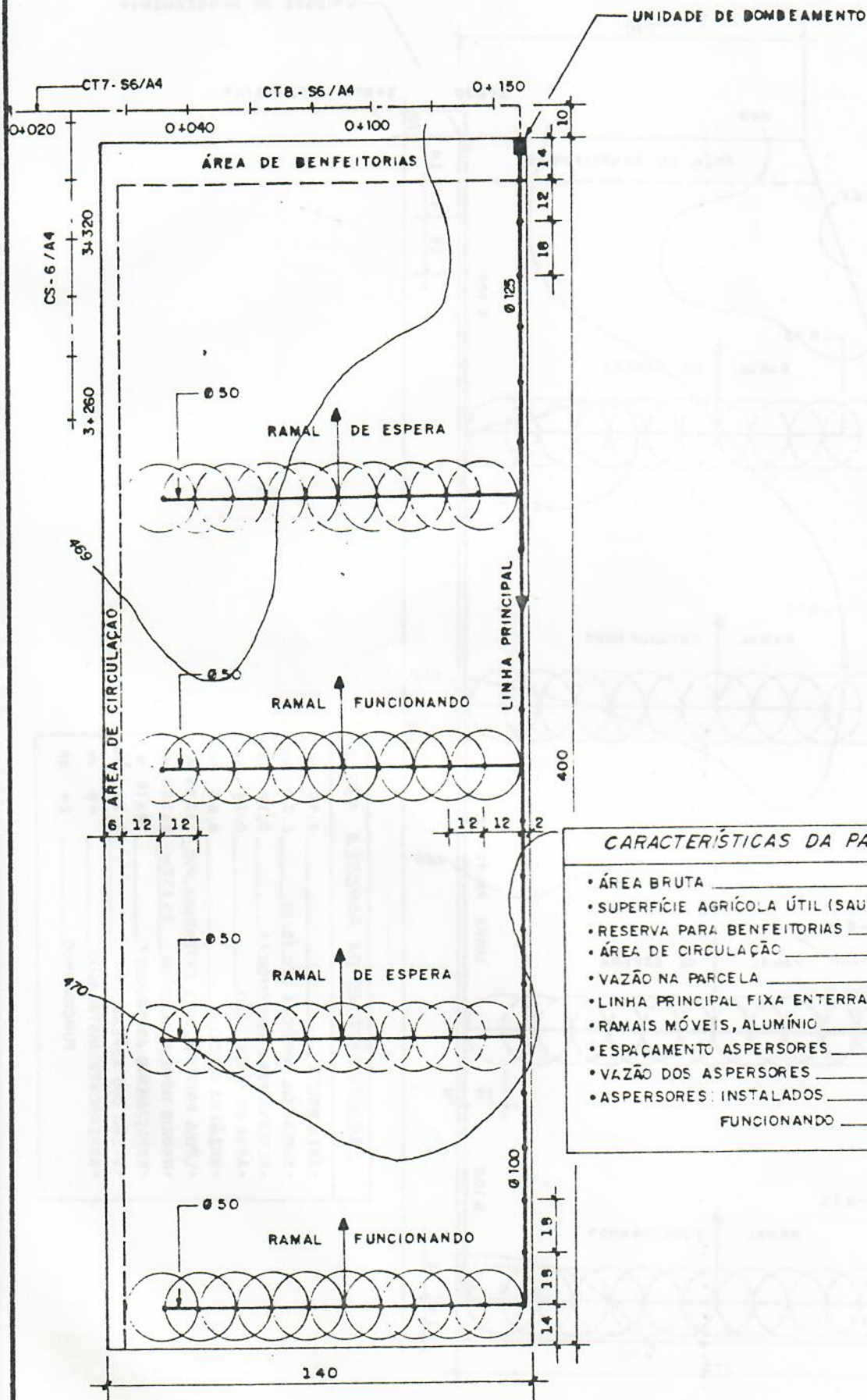
Fig. 100 REDE PARCELAR
