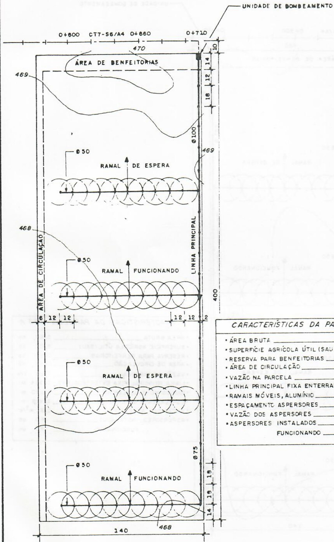
Fig. 22 REDE PARCELAR
