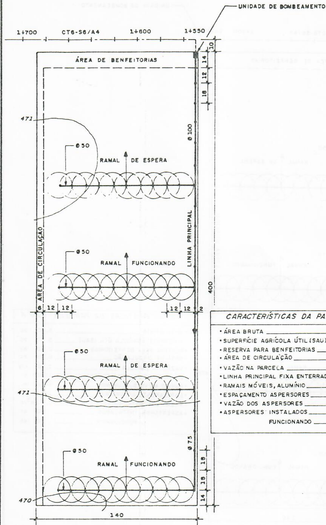
Fig.819 REDE PARCELAR
