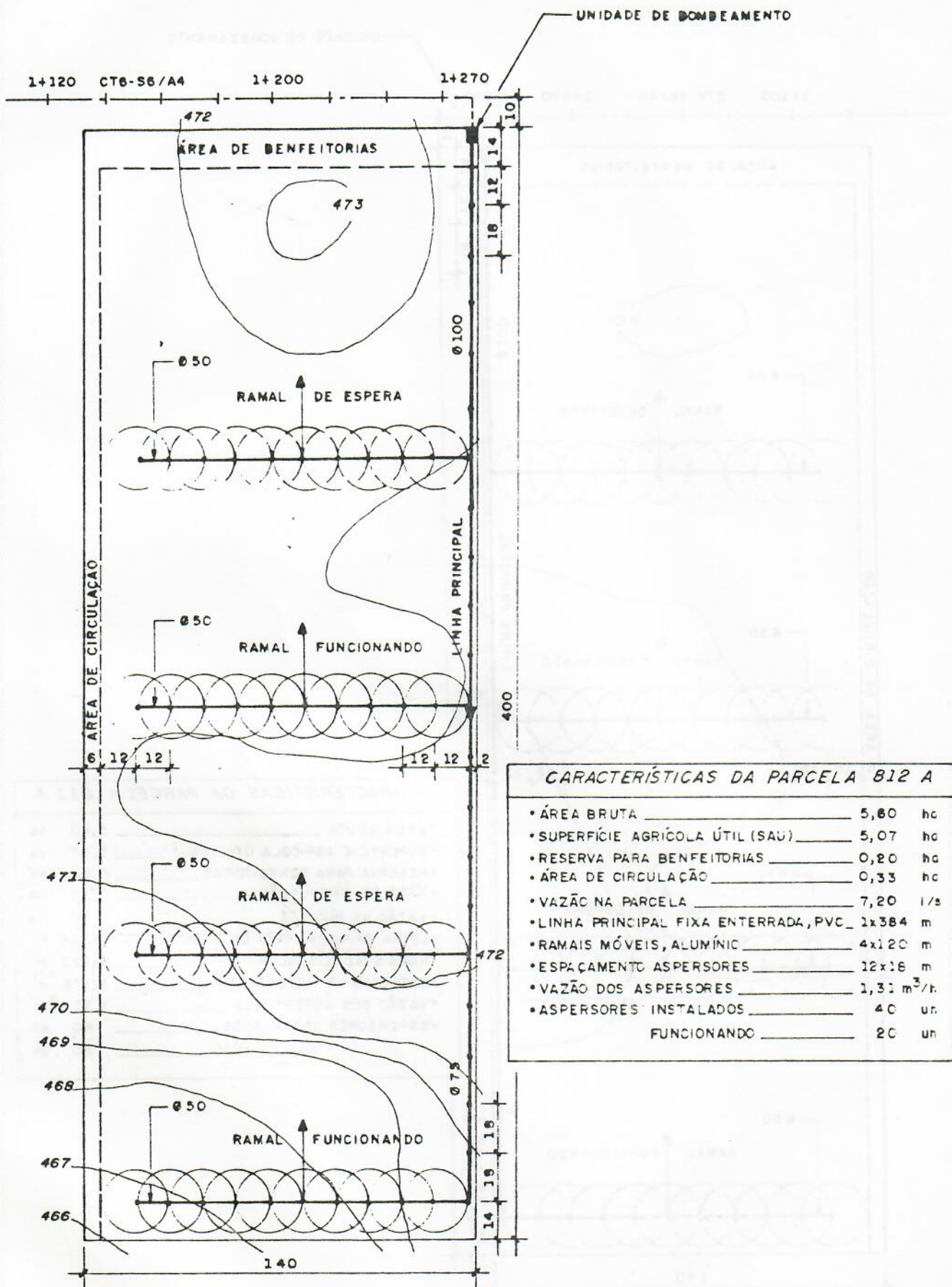
Fig. 512 REDE PARCELAR
