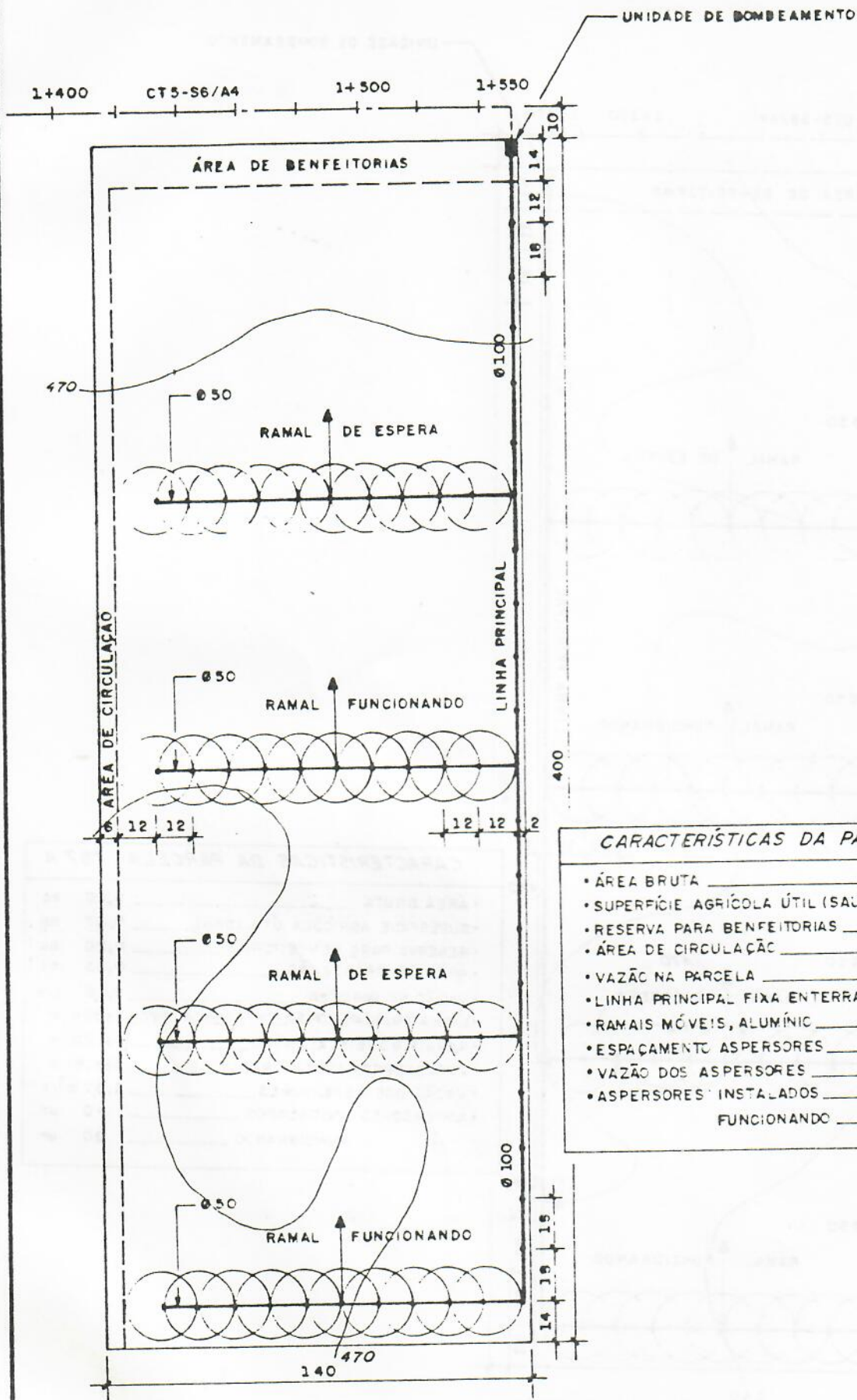
Fig. 188 REDE PARCELAR
