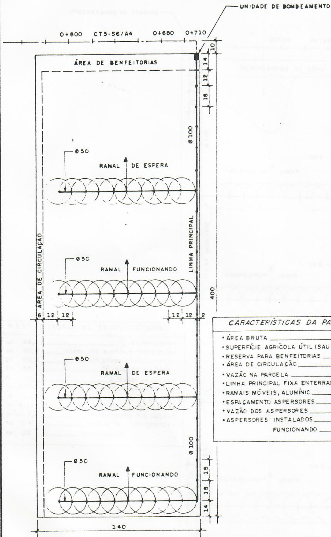
Fig. 216 REDE PARCELAR
