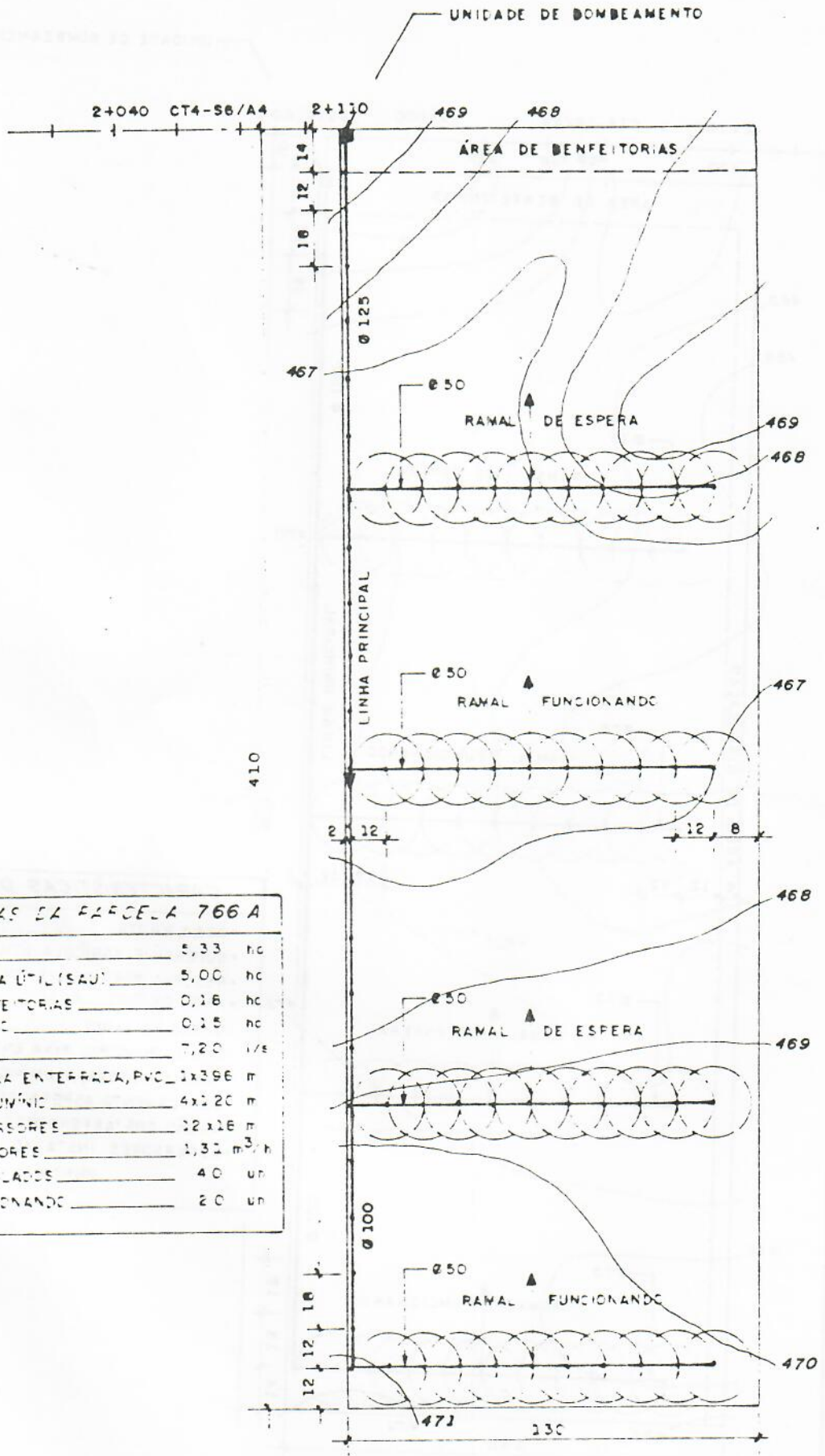
Fig. 500 REDE PARCELAR
