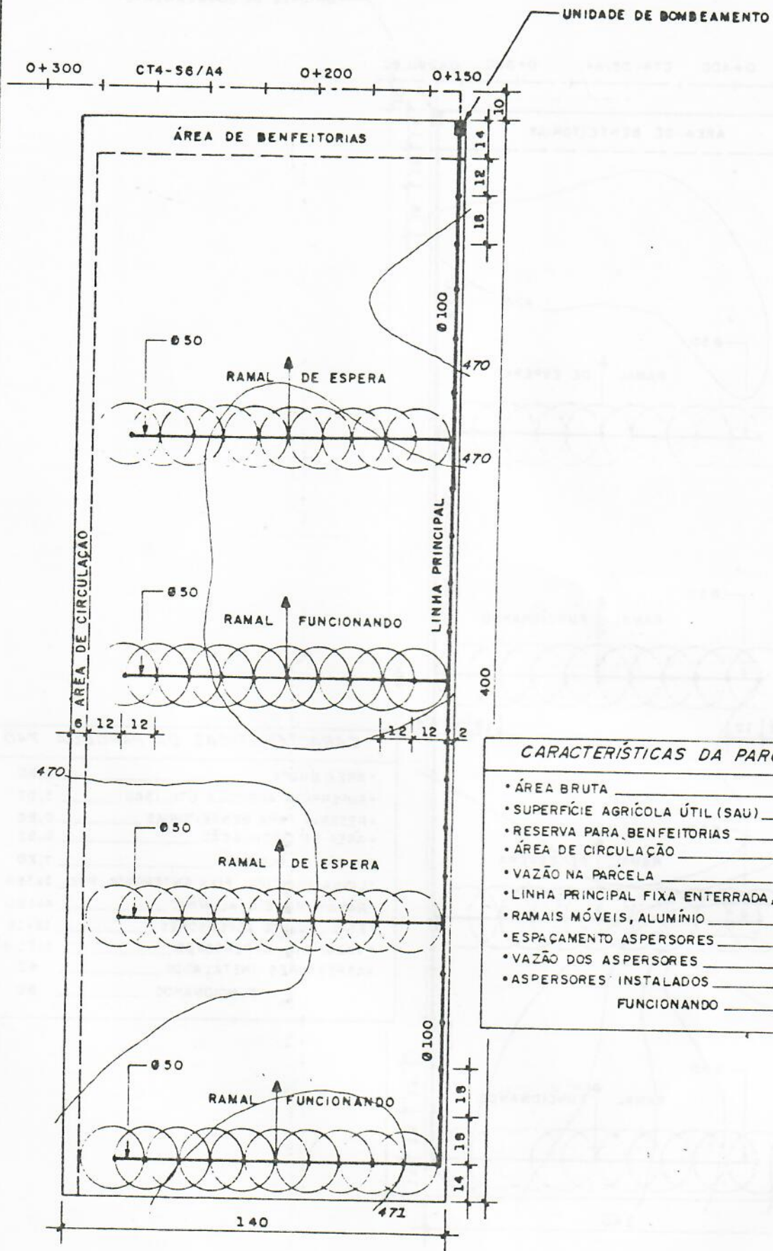
Fig. 738 REDE PARCELAR
