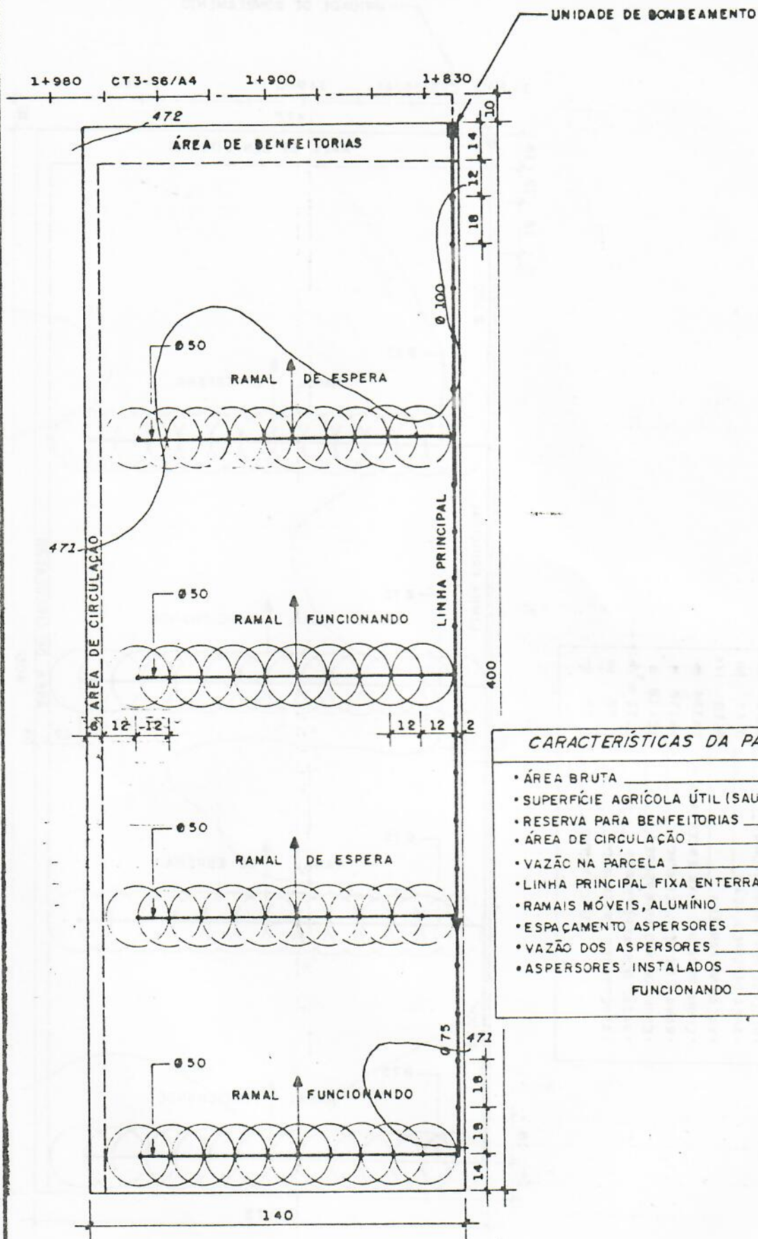
Fig. 733 REDE PARCELAR
