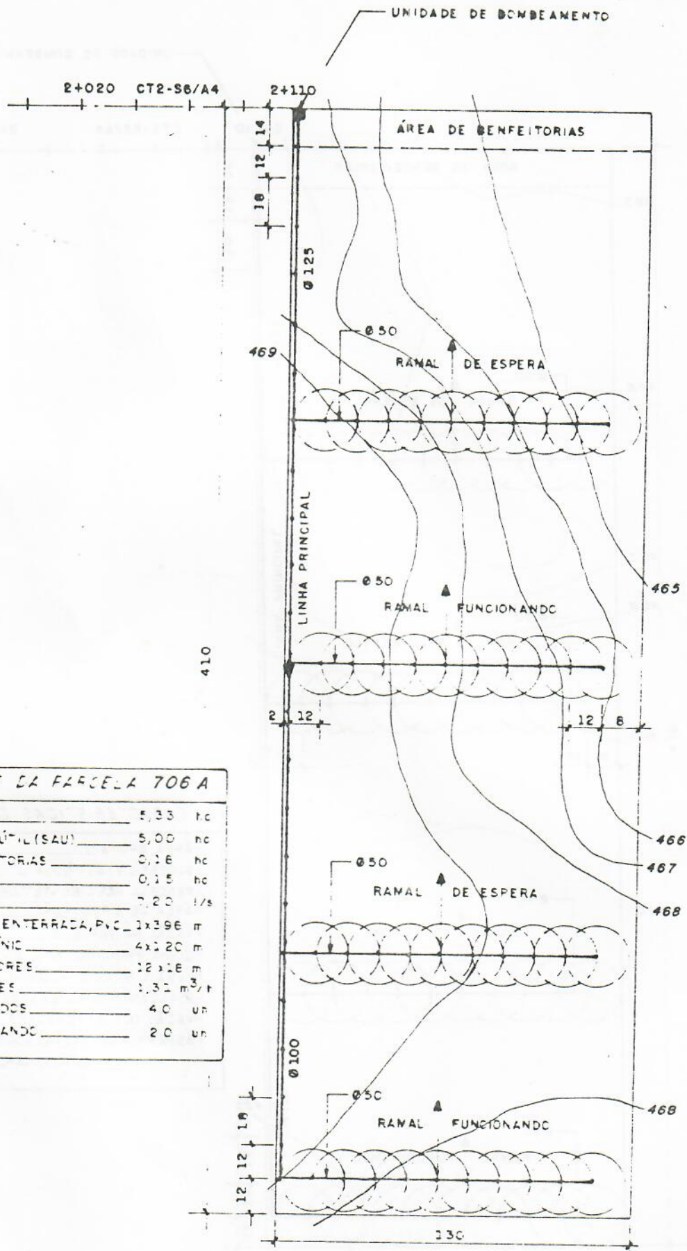
Fig. 706 REDE PARCELAR
