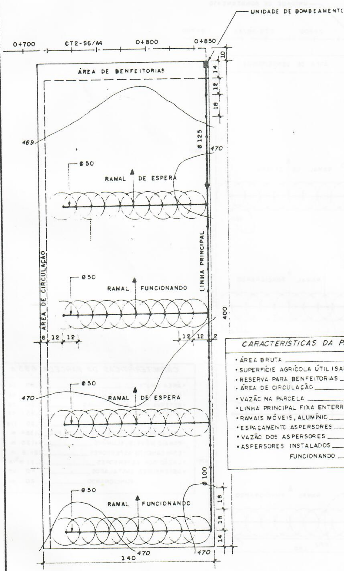
Fig. 050 REDE PARCELA
