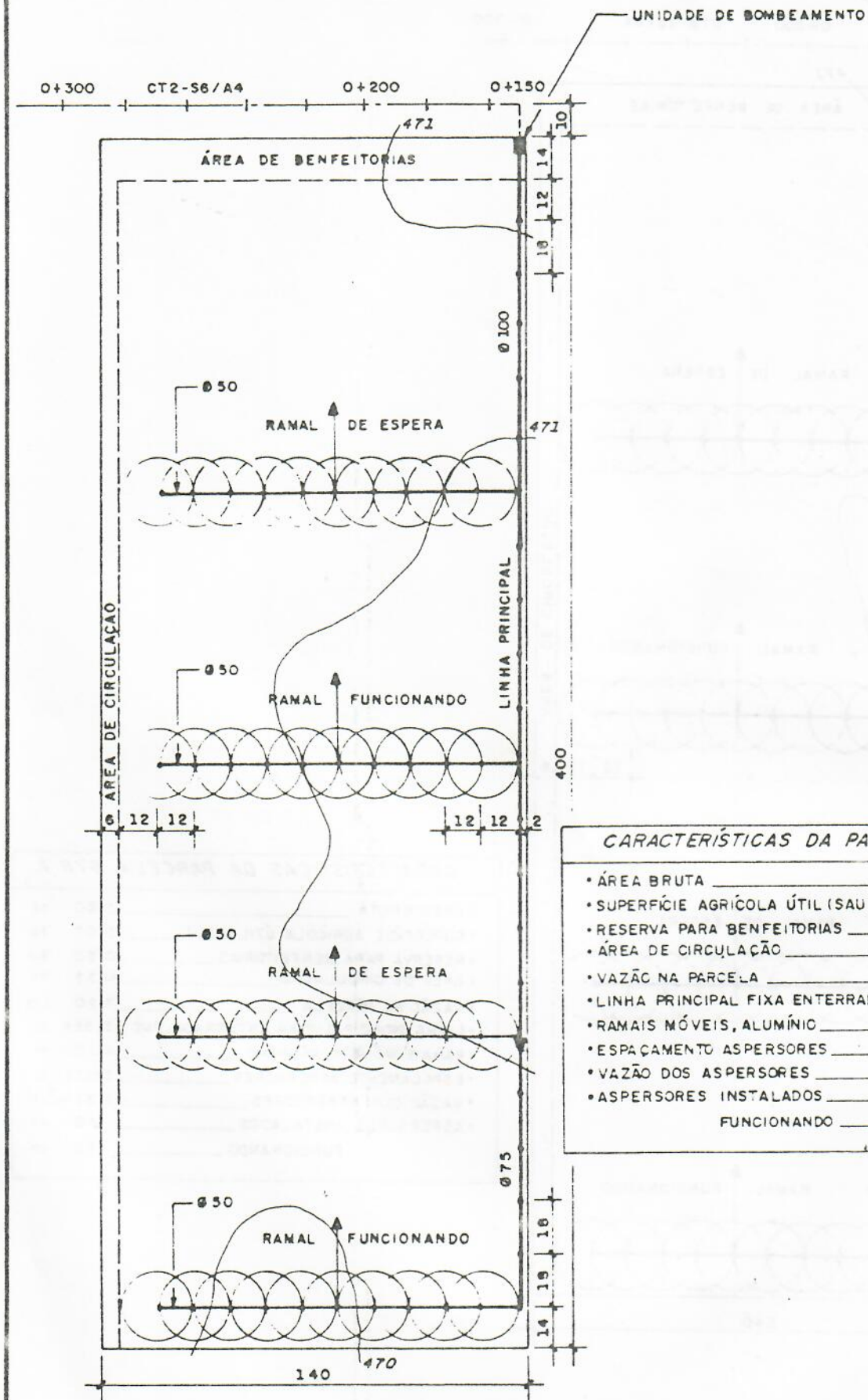
Fig. 67 REDE PARCELAR
