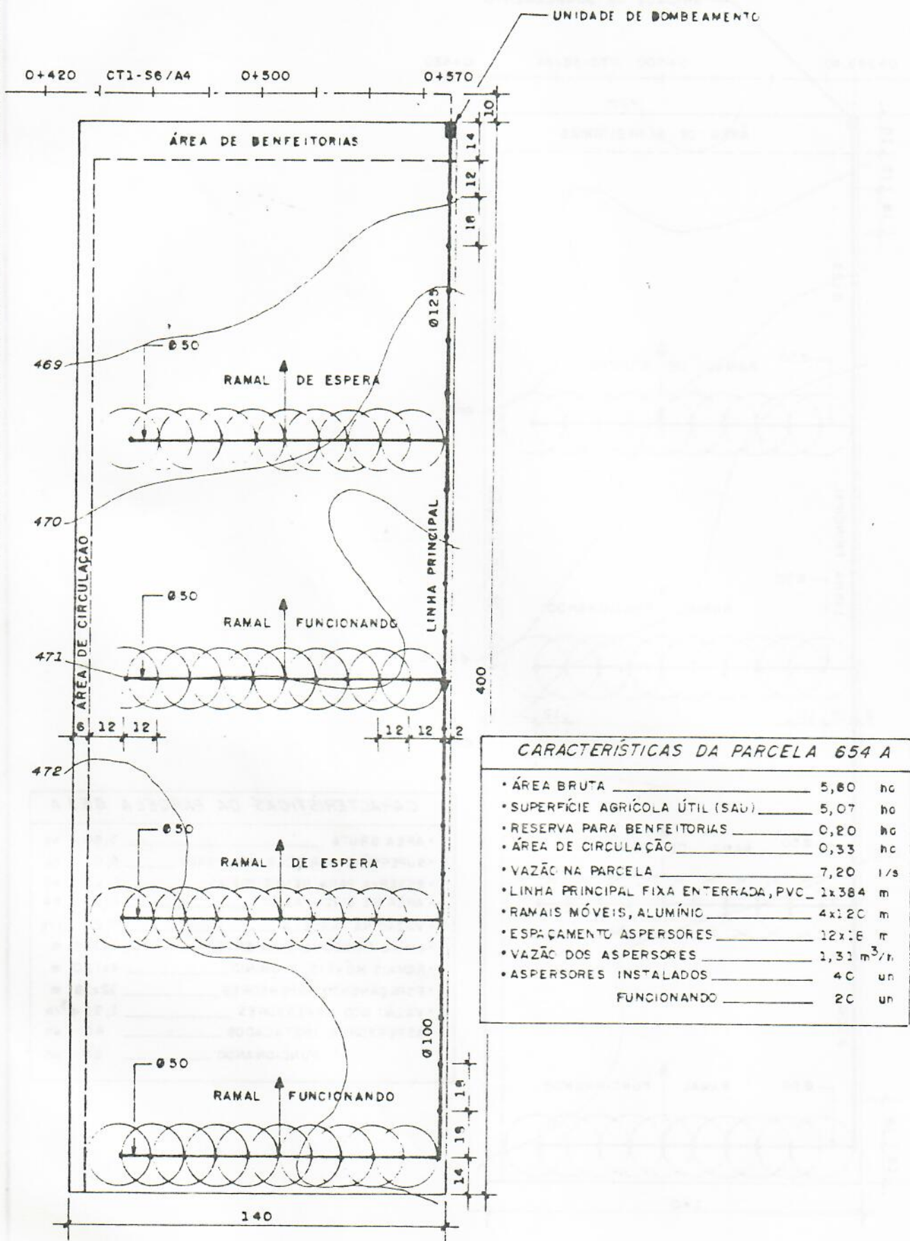
Fig. 201 REDE PARCELAR
