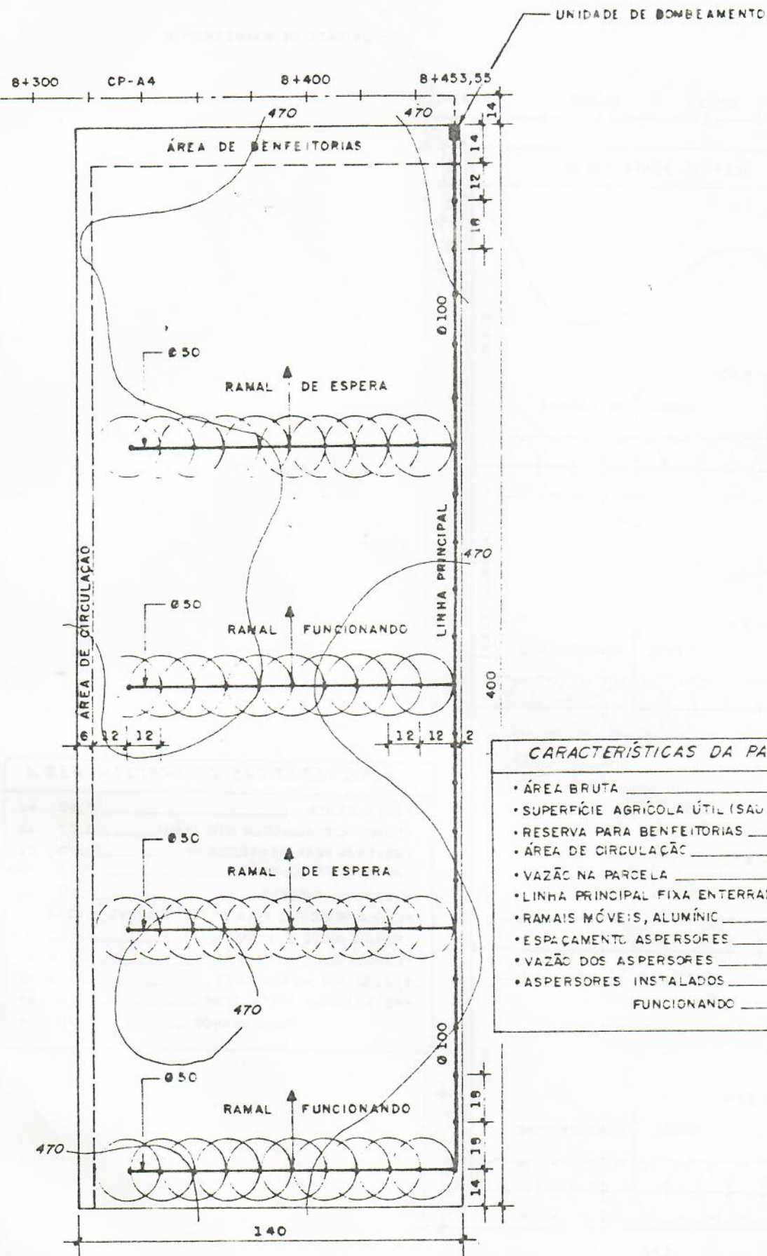
Fig. 640 REDE PARCELAR
