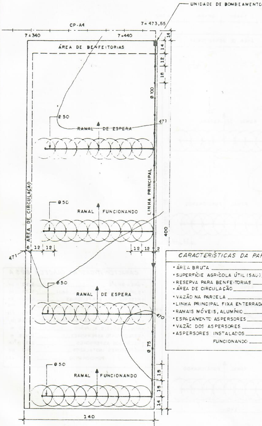
Fig. 626 REDE PARCELAR
