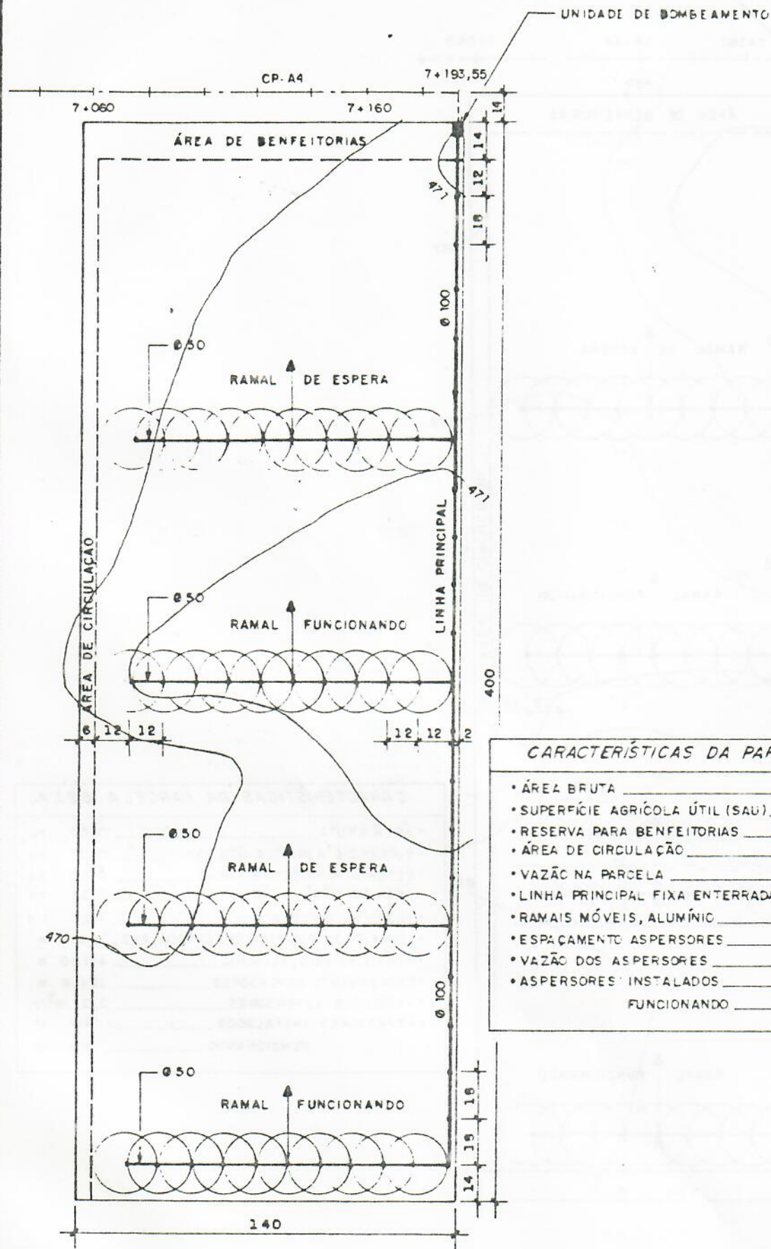
Fig. 622 REDE PARCELAR
