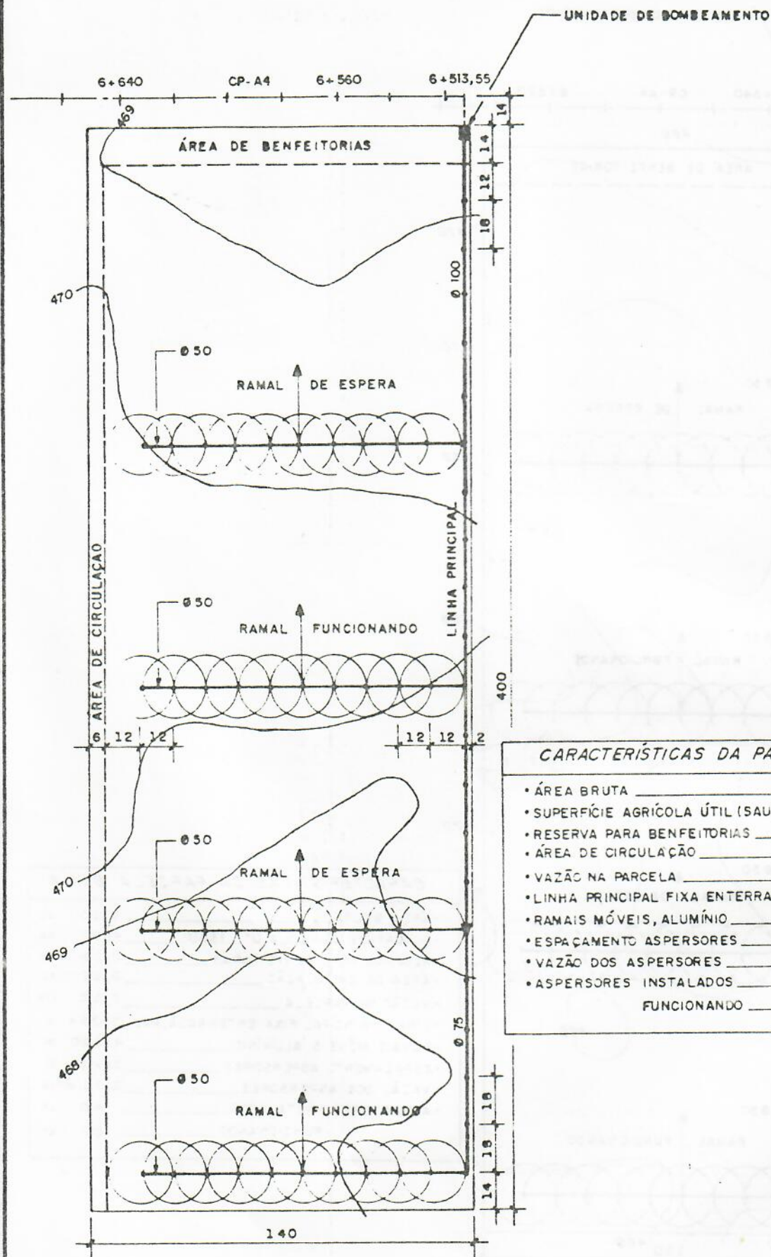
Fig. 23 REDE PARCELAR
