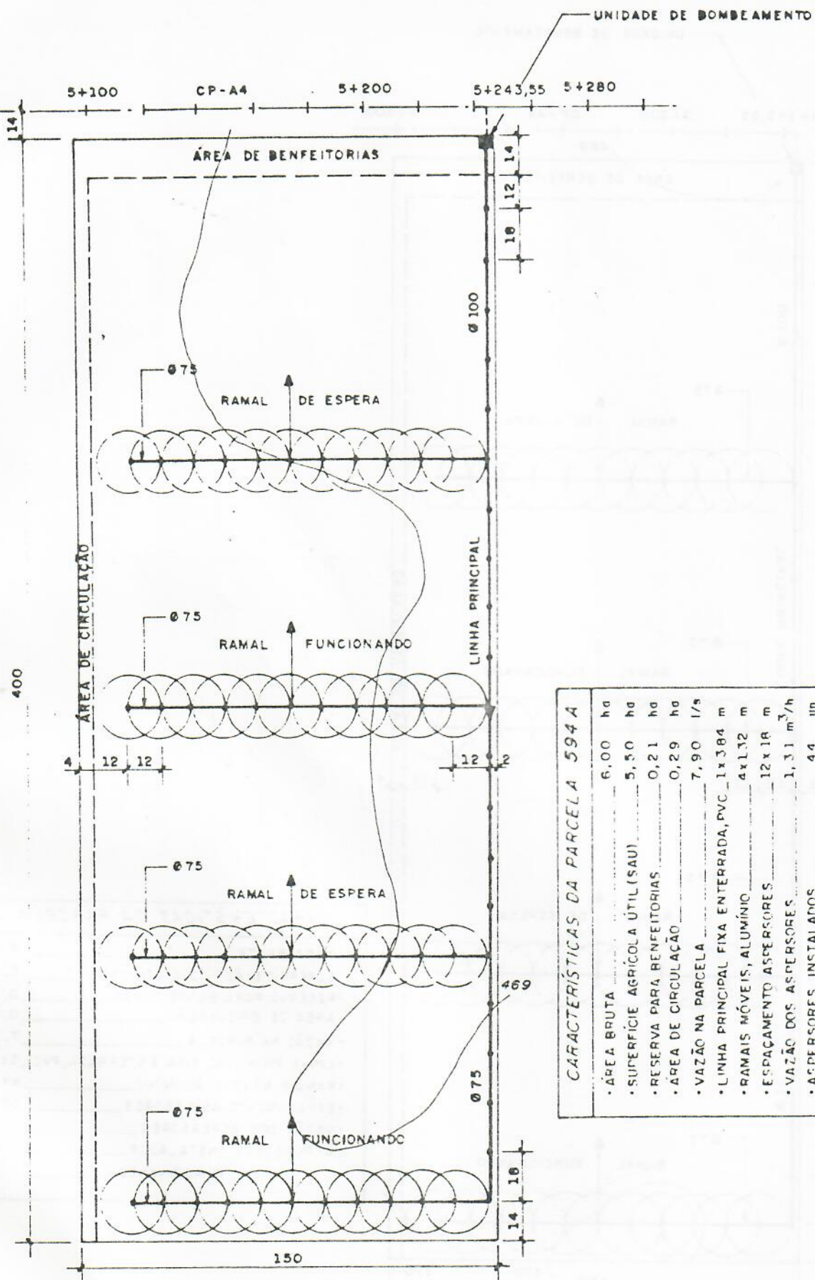
Fig. 5.4 REDE PARCELAR
