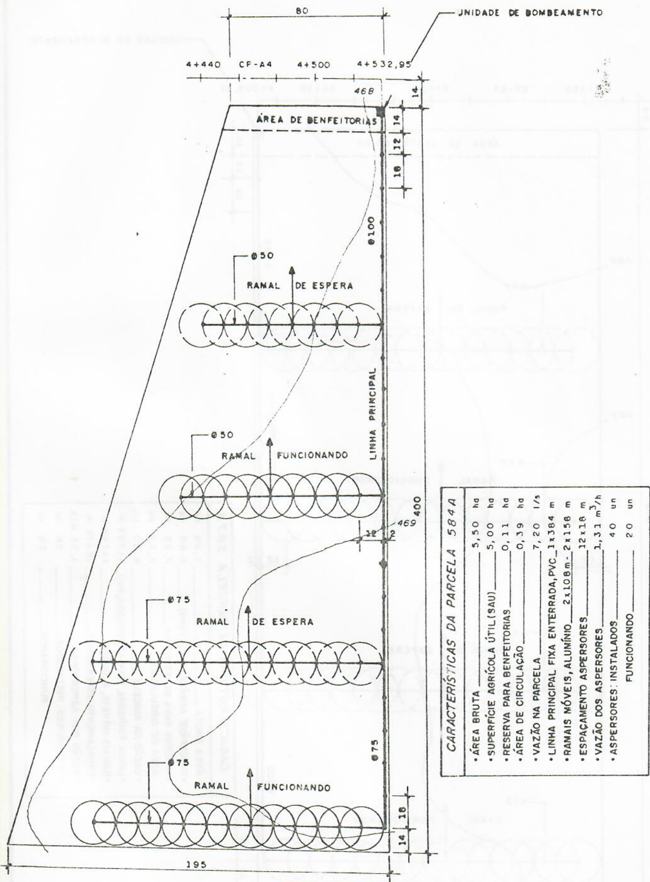
Fig. 1 - REDE PARCELAR
