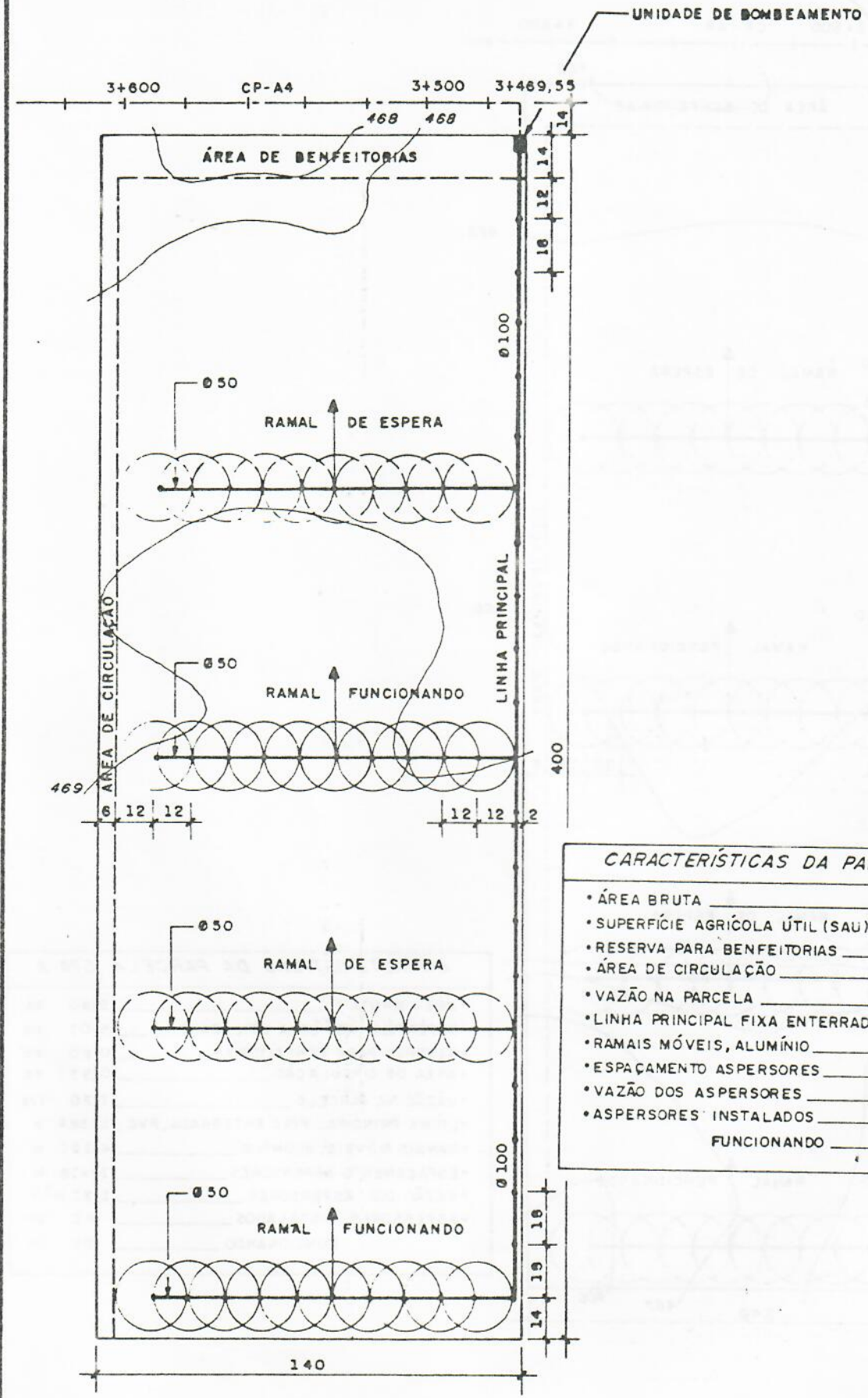
Fig. 573 REDE PARCELAR
