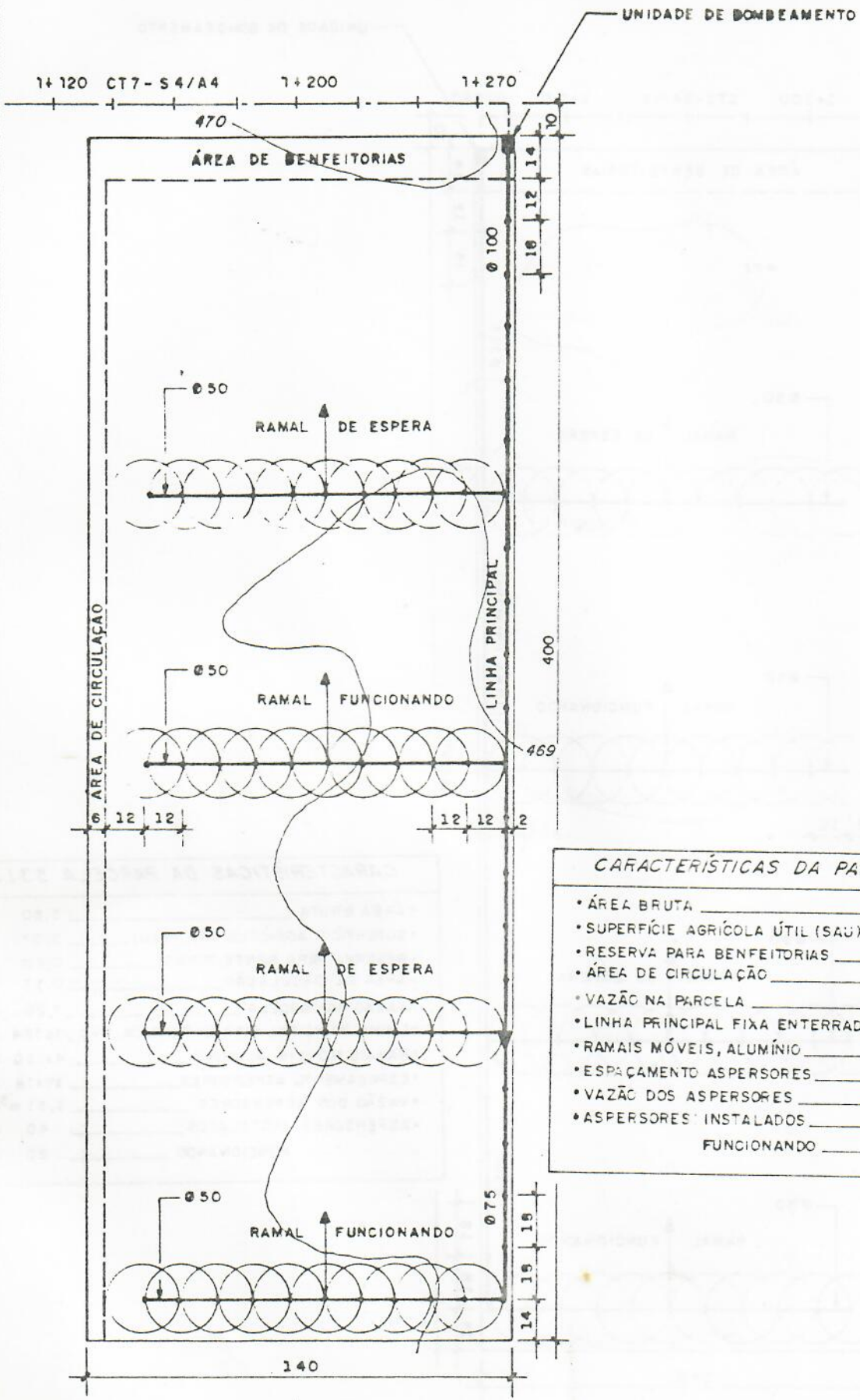
Fig. 5.2 REDE PARCELAR
