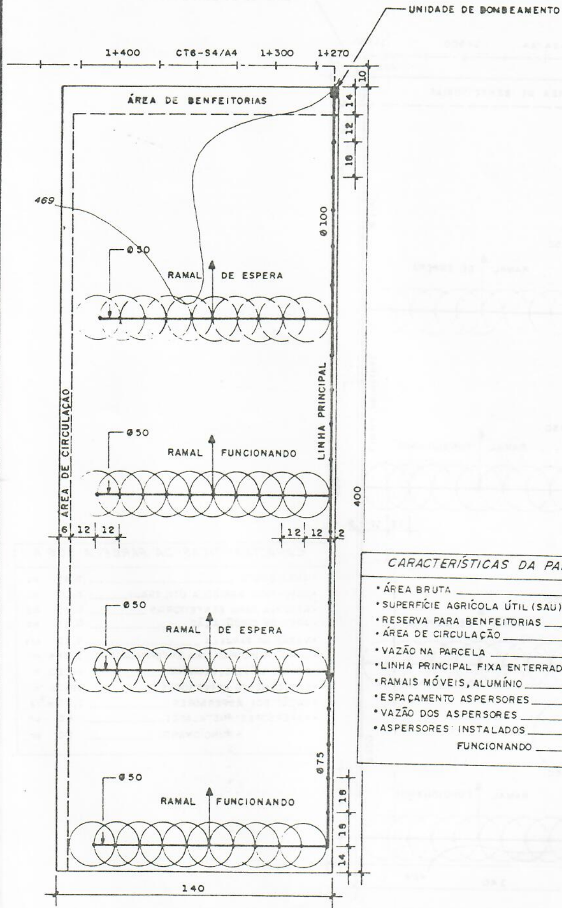
Fig. 505 REDE PARCELAR
