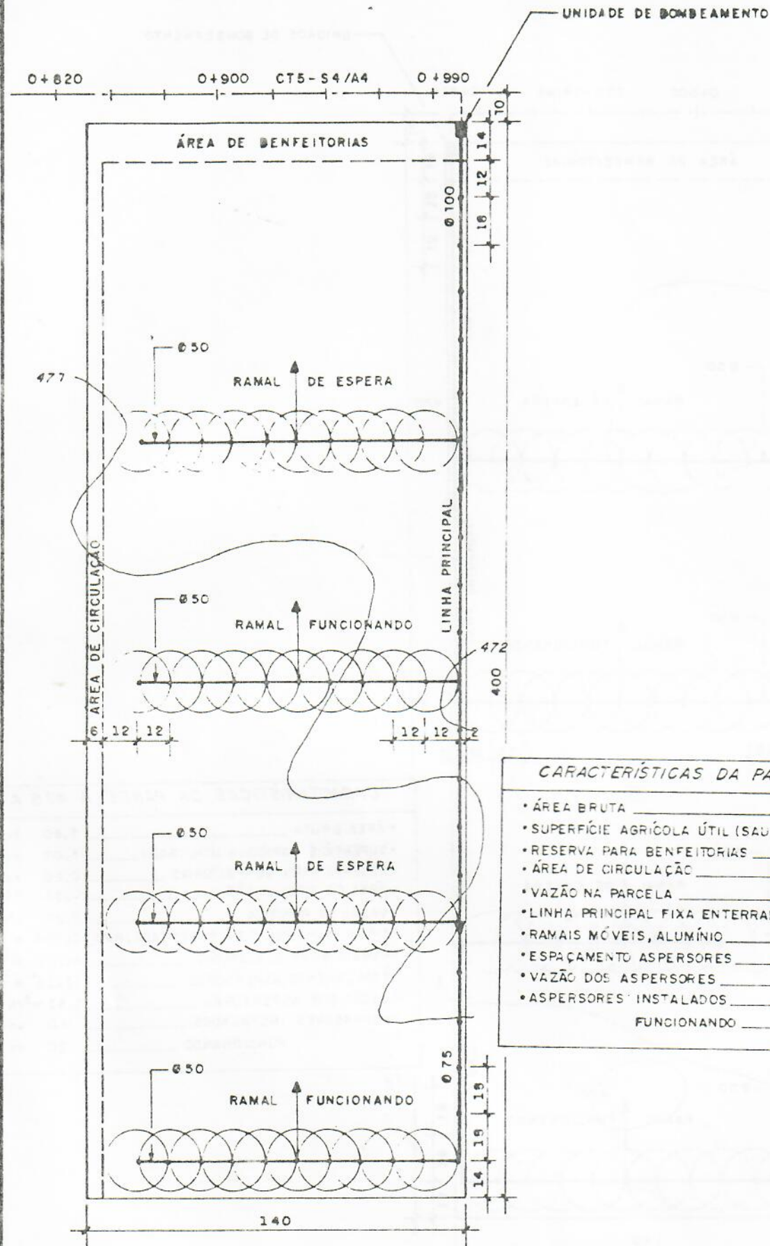
Fig. 476 REDE PARCELAR
