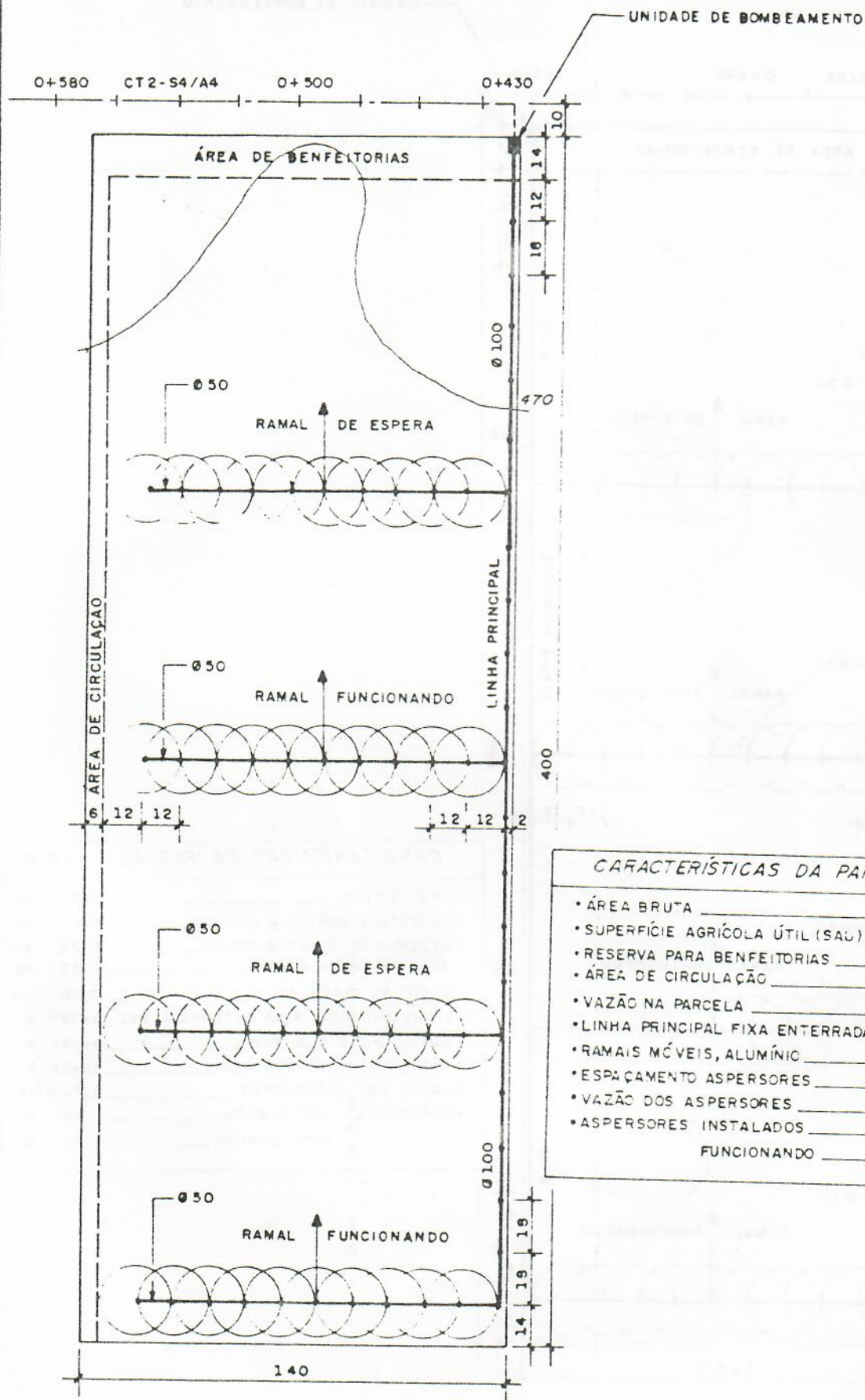
Fig. 412 REDE PARCELAR
