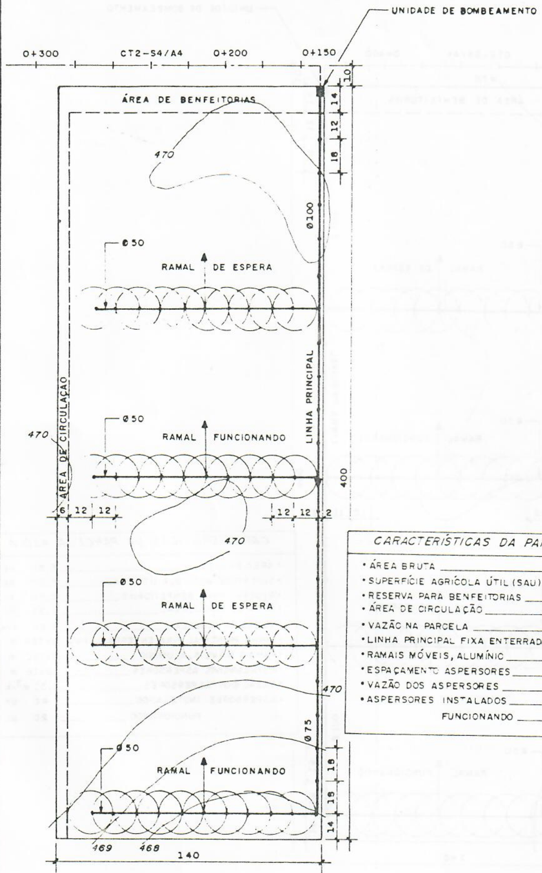
Fig. 602 REDE PARCELAR
