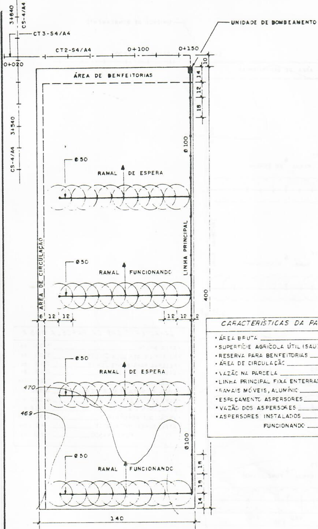
Fig. 406 REDE PARCELAR
