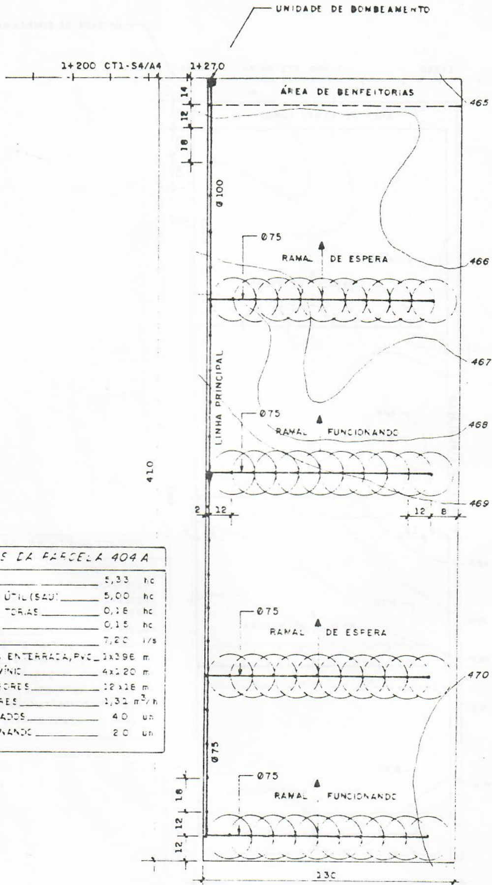
Fig. 4.2 REDE PARCELAR
