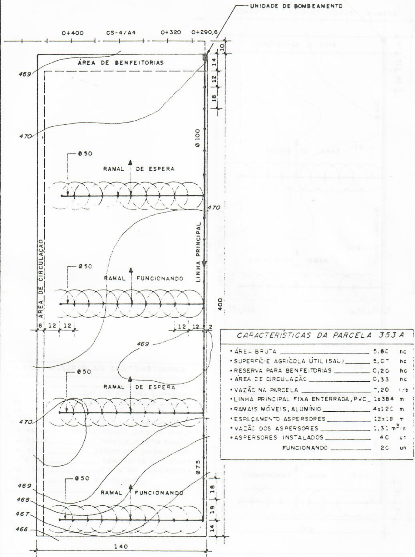
Fig. 222 REDE PARCELAR
