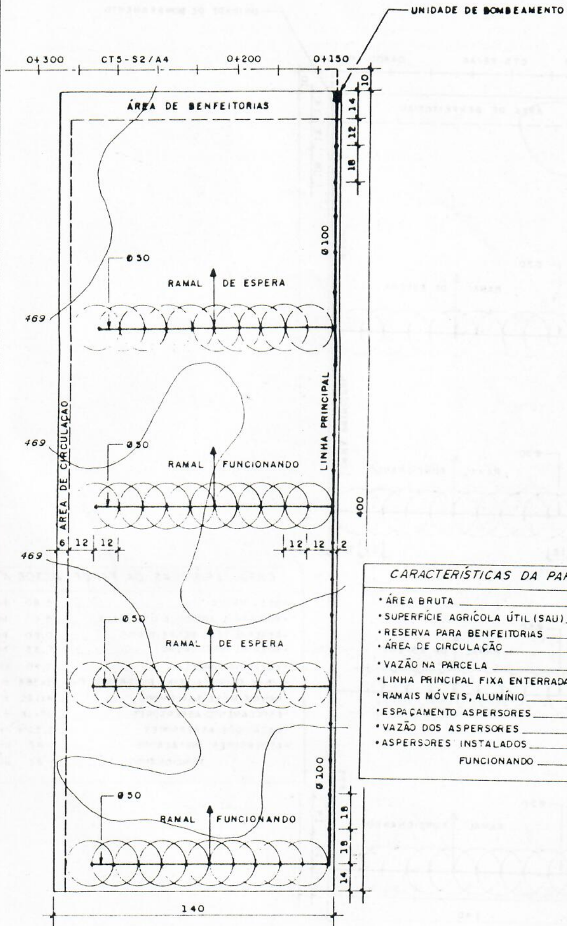
Fig. 303 REDE PARCELAR
