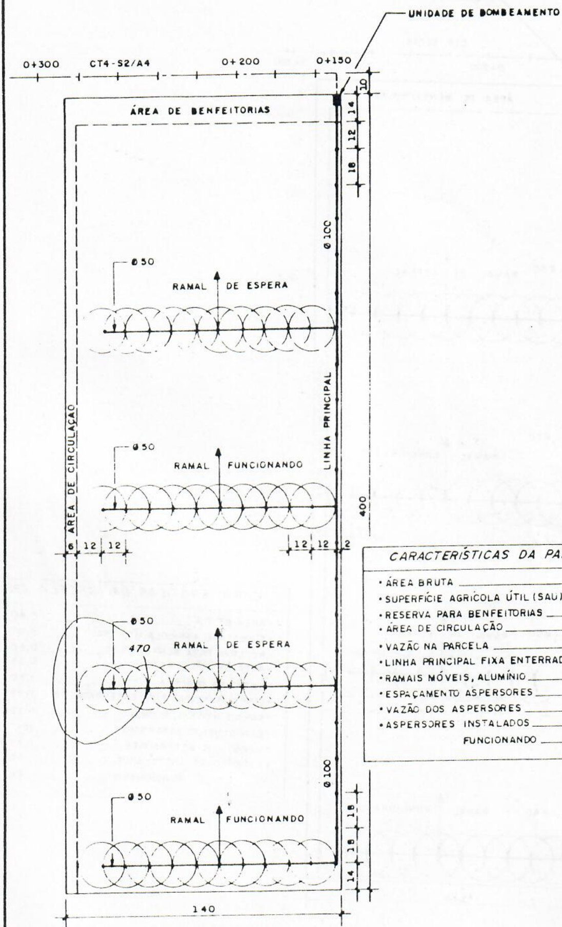
Fig. 288 REDE PARCELAR
