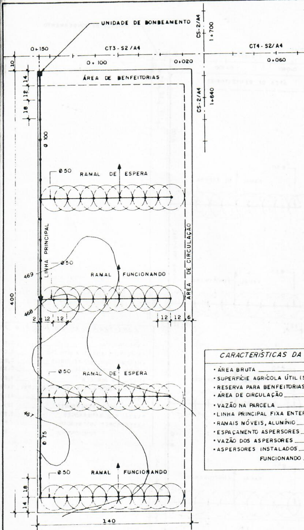
Fig. 369 REDE PARCELAR
