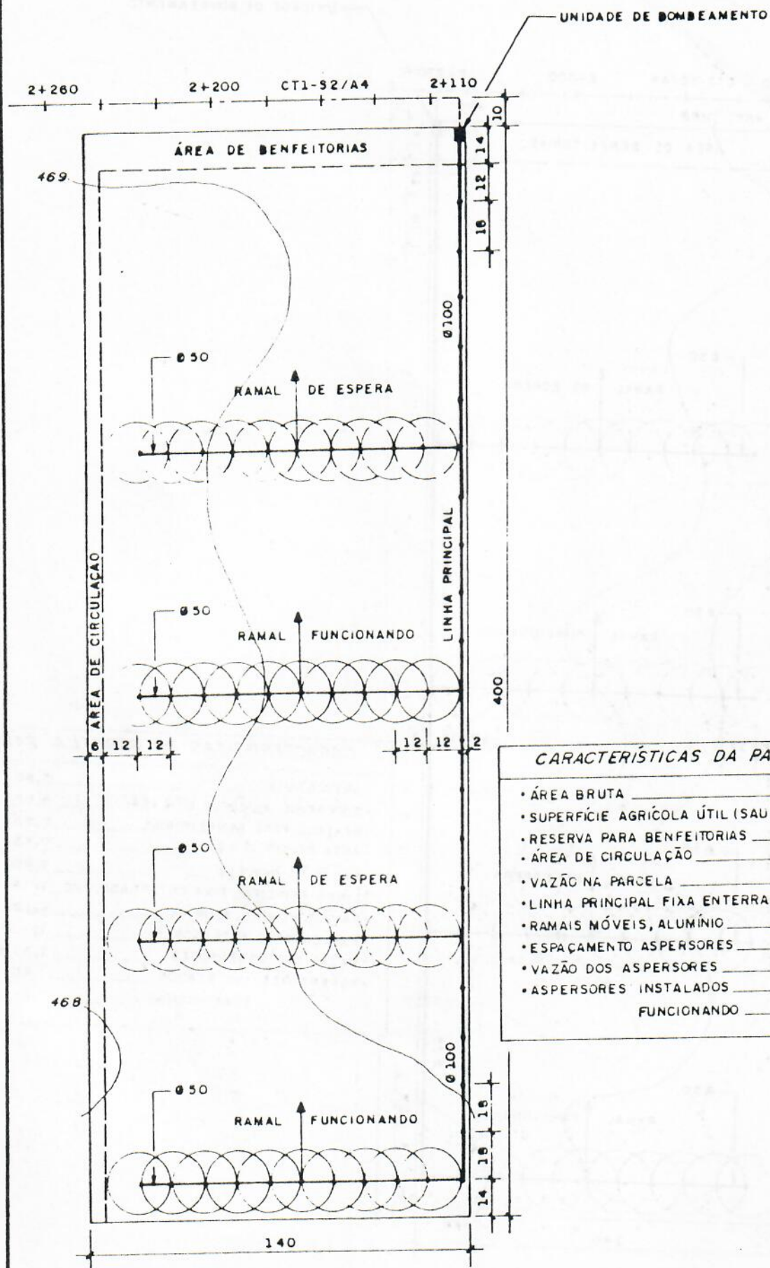
Fig. 247 REDE PARCELAR
