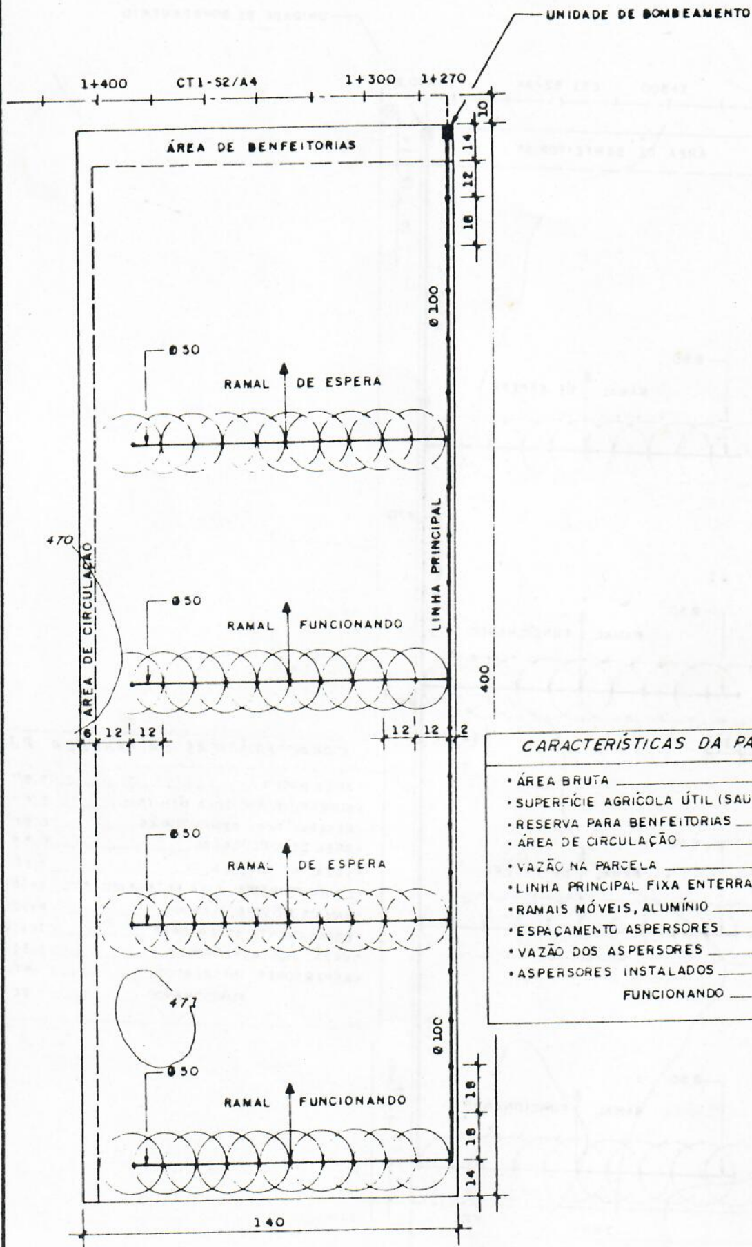
Fig. 235 REDE PARCELAR
