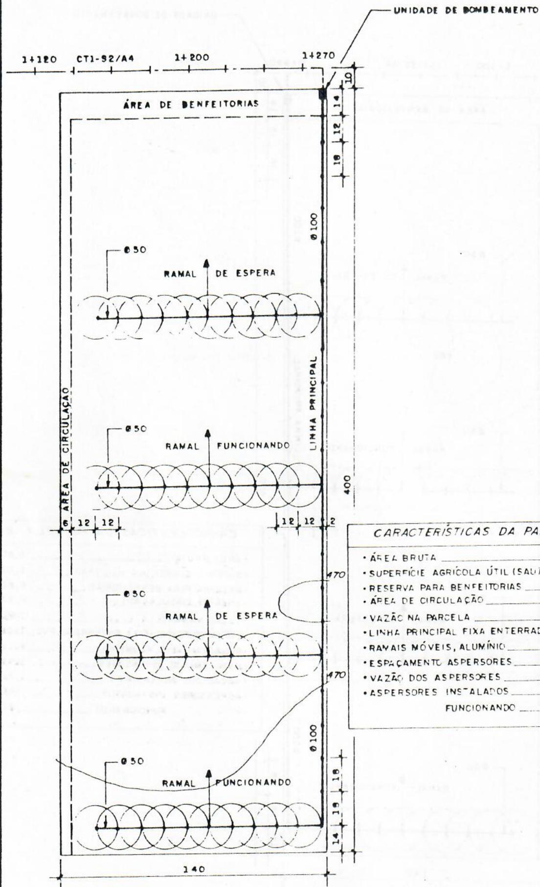
Fig. 22. REDE PARCELAR
