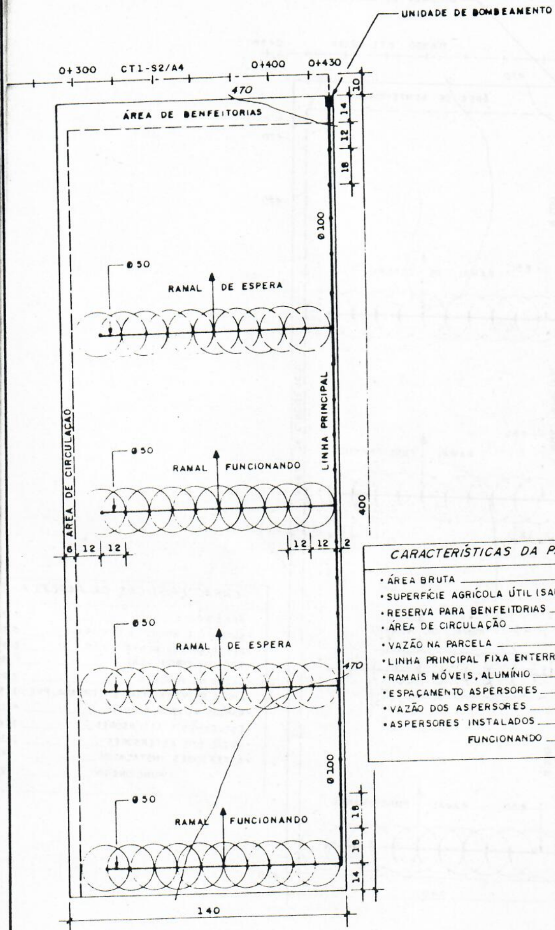
Fig. 221 REDE PARCELAR
