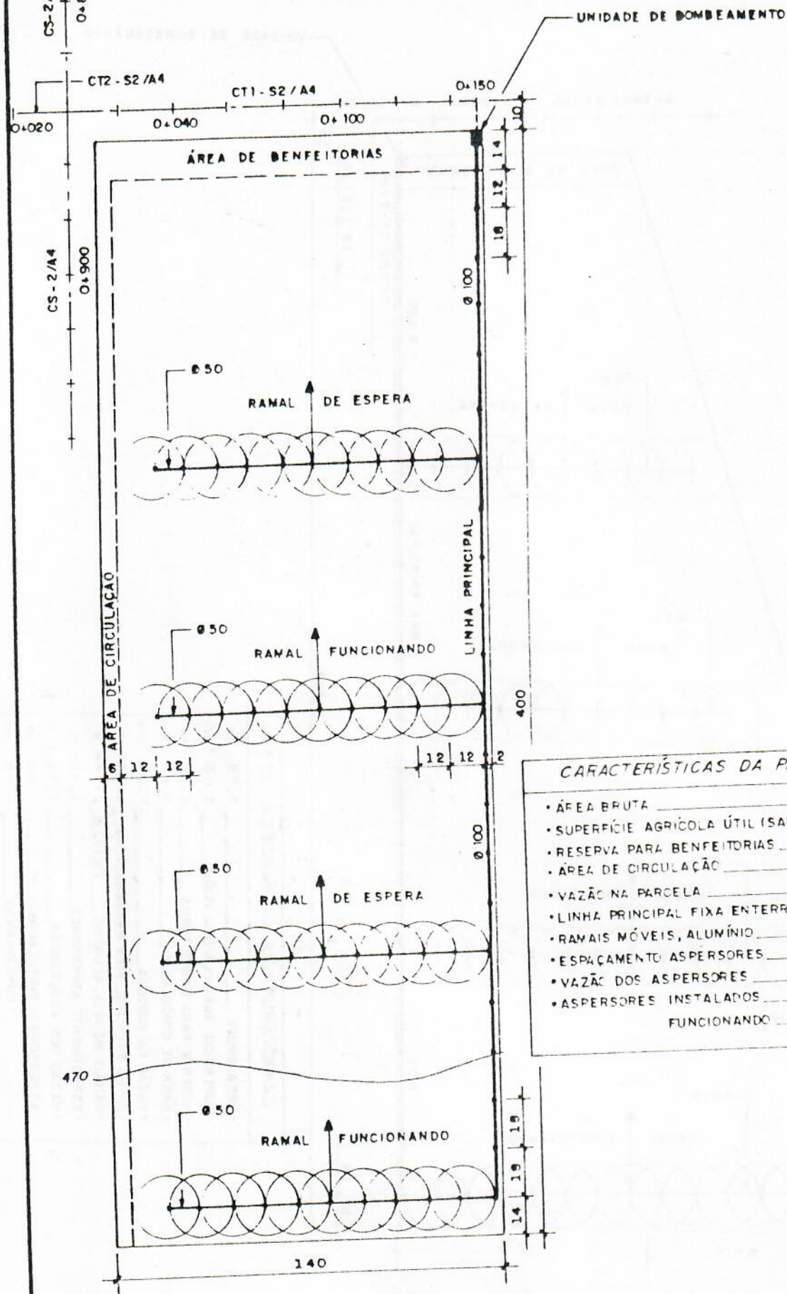
Fig. 216 REDE PARCELAR
