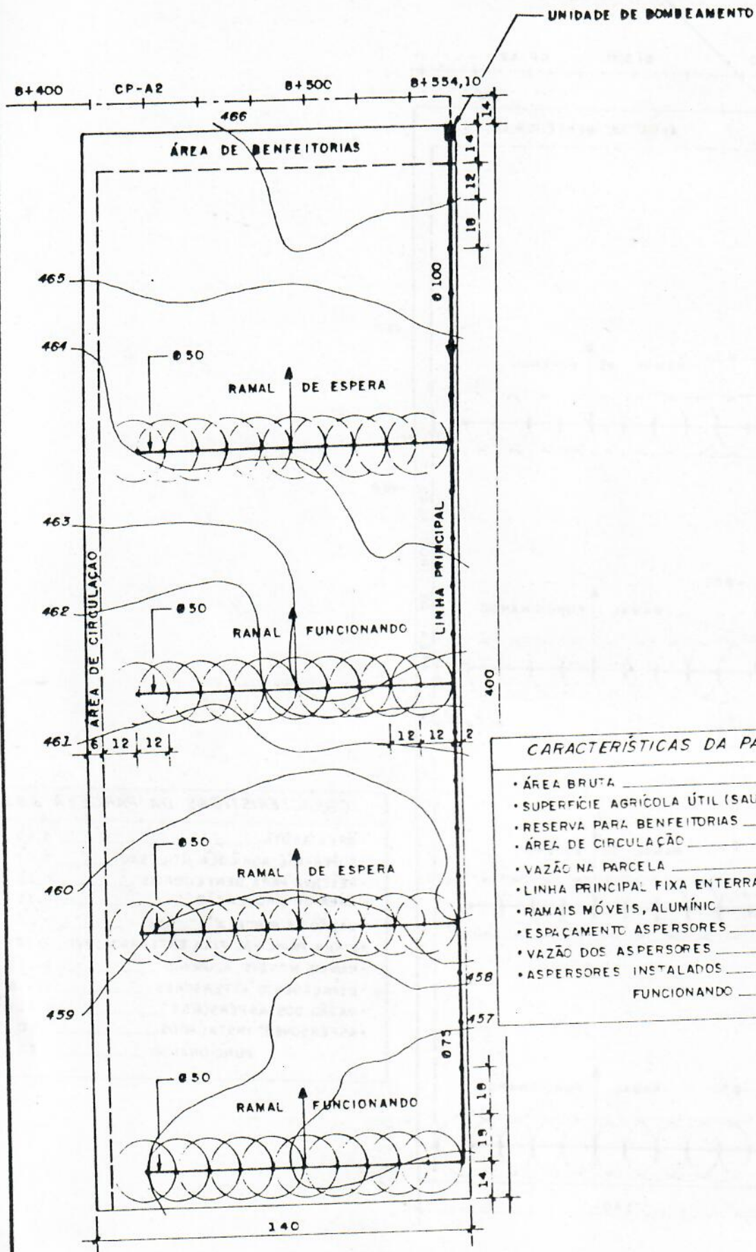
Fig. 15- REDE PARCELAR
