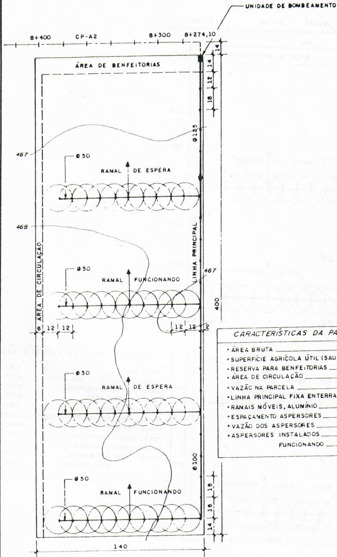
Fig. 181 REDE PARCELAR
