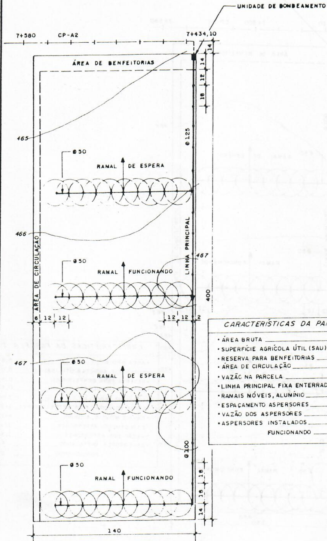
Fig. 169 REDE PARCELAR
