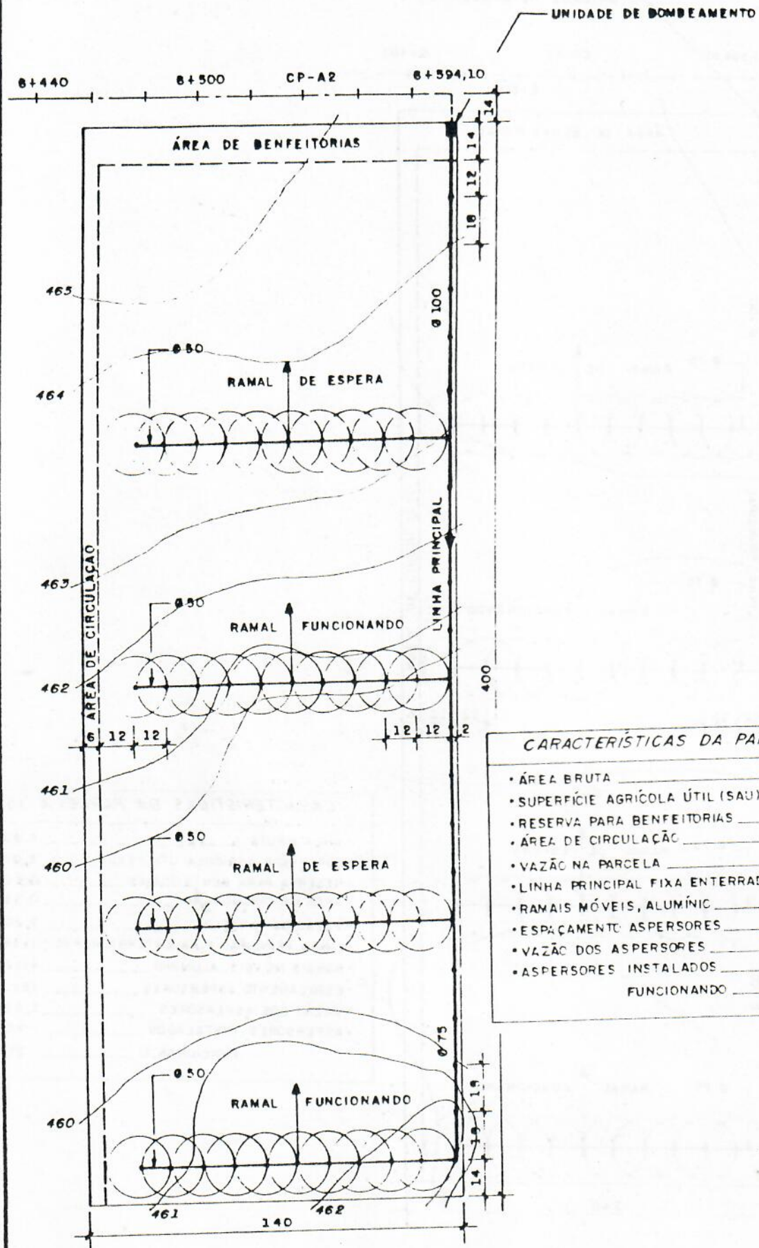
Fig. 10c REDE PARCELAR
