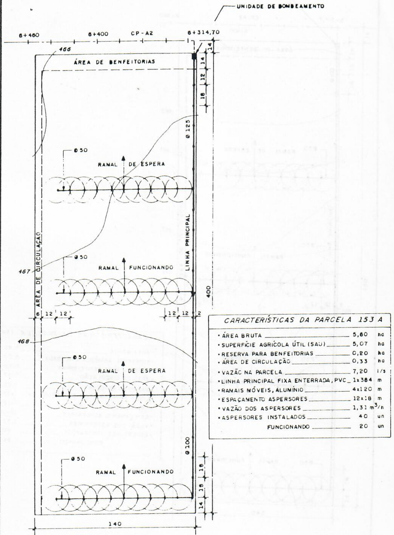
Fig.153 REDE PARCELAR
