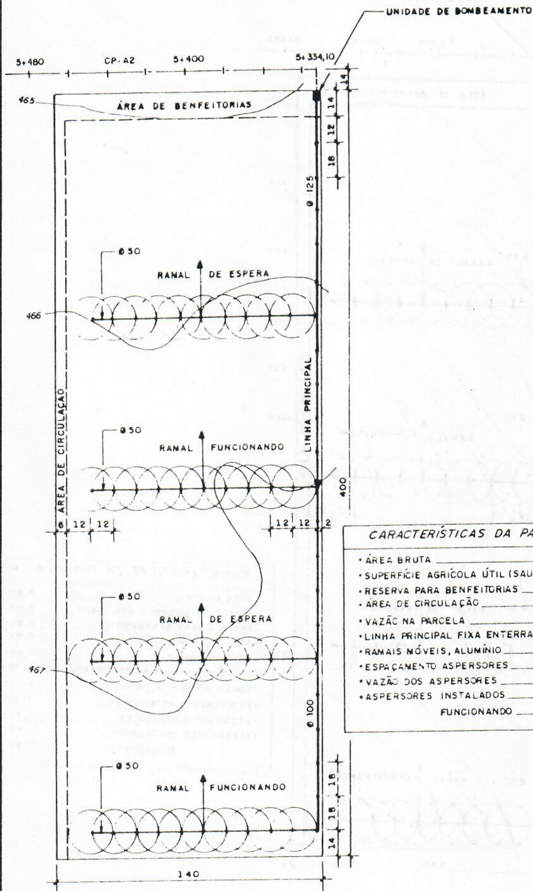
Fig. 189 REDE PARCELAR
