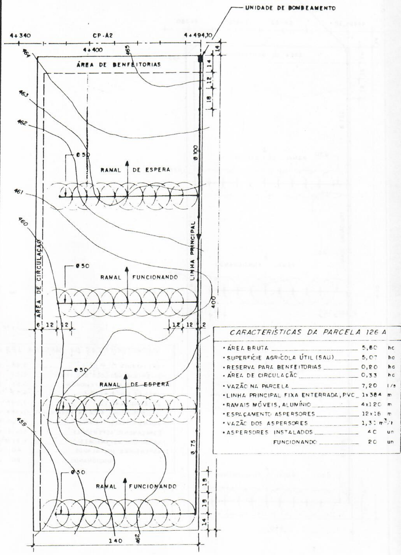
Fig. 102 REDE PARCELAR
