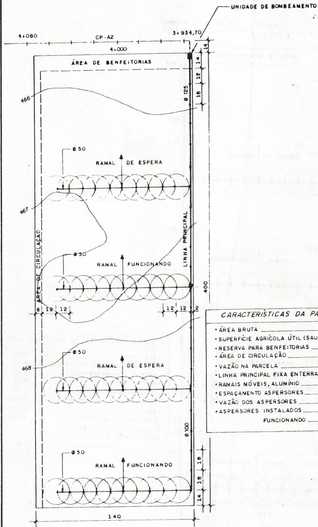
Fig. 200 REDE PARCELAR
