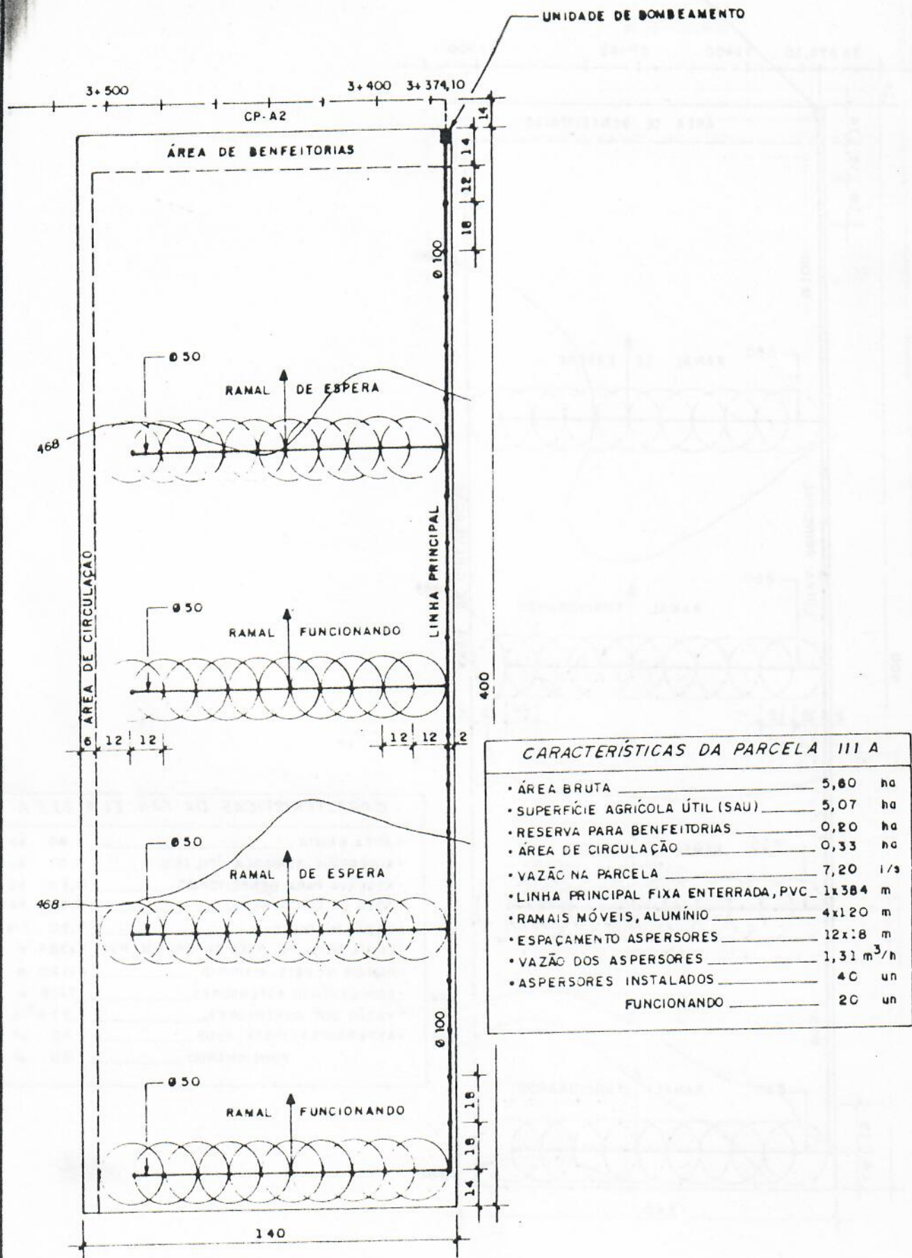
Fig. 111 REDE PARCELAR
