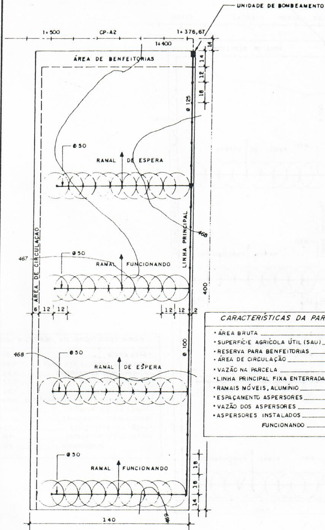
Fig. 51 REDE PARCELAR
