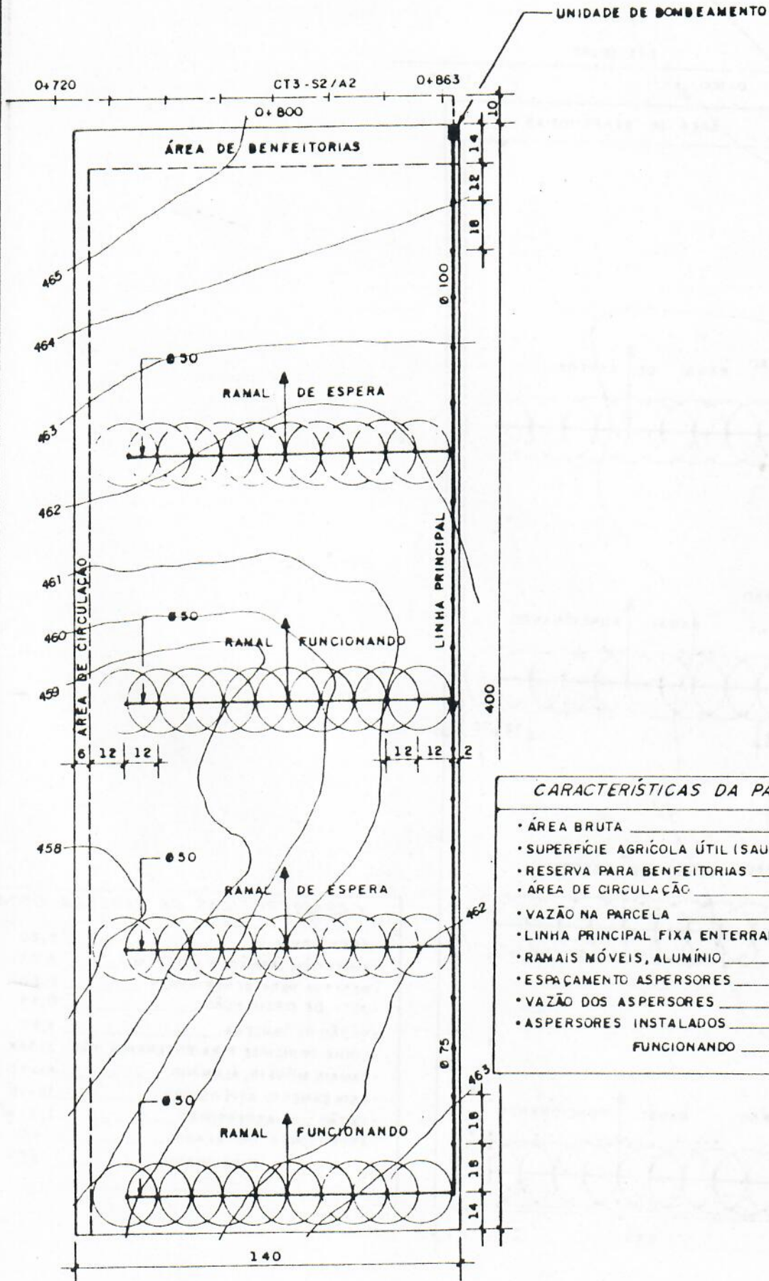
Fig. 49 REDE PARCELAR
